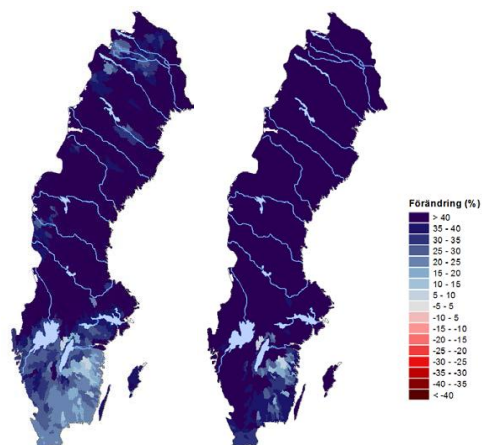
Figur 1d. Förändring (%) av vattentillgång för vintern (december, januari och februari) mellan referensperioden 1963-1992 och perioden 2069-2098 för RCP4.5 till vänster och RCP8.5 till höger 5 .
